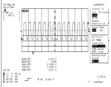
Ref.4 ITU 656 Clock out : IC200, #83
