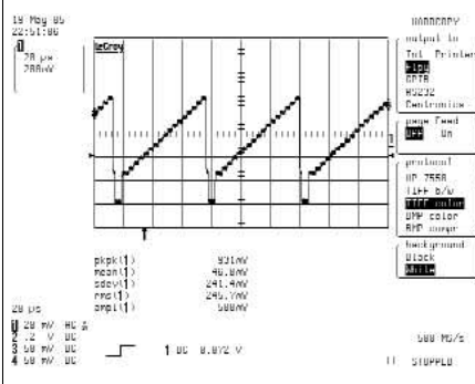
Ref.3 Y separated output : IC300, #96
