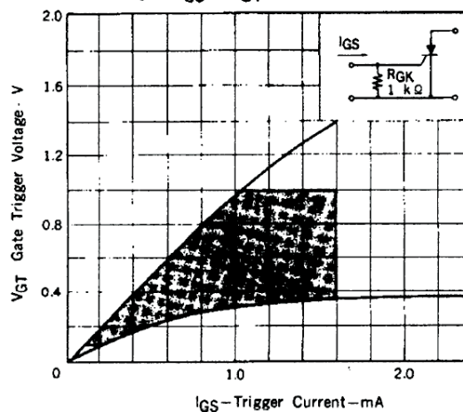
Fig. 4 I_{GS} - V_{GT} DISTRIBUTION
